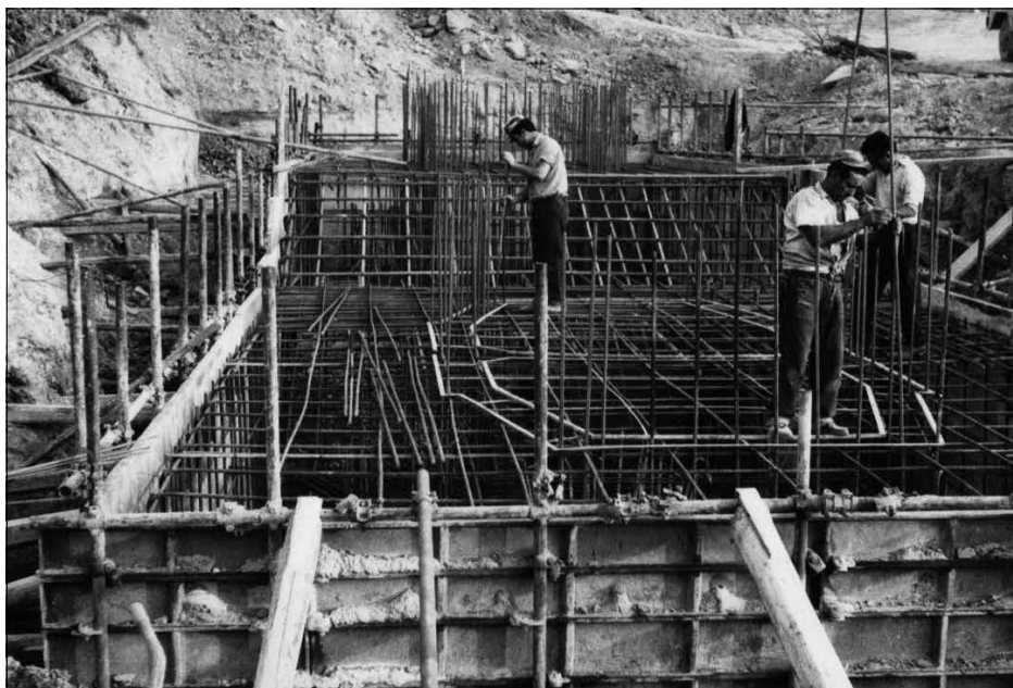
L'armatura di una zattera di fondazione
